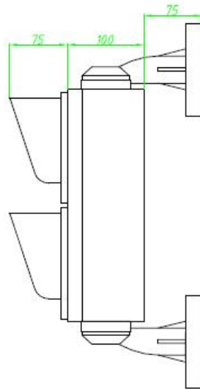
右视图
