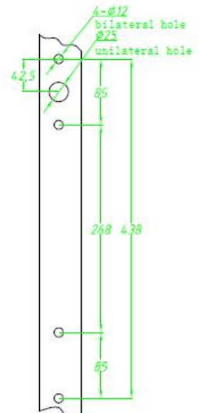
灯杆钻孔图
