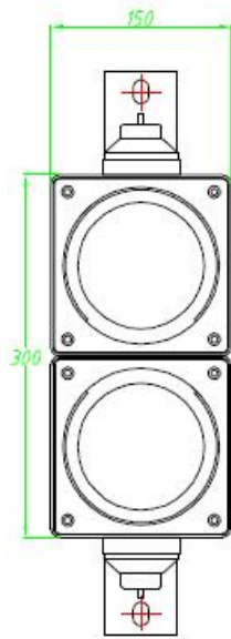
主视图
